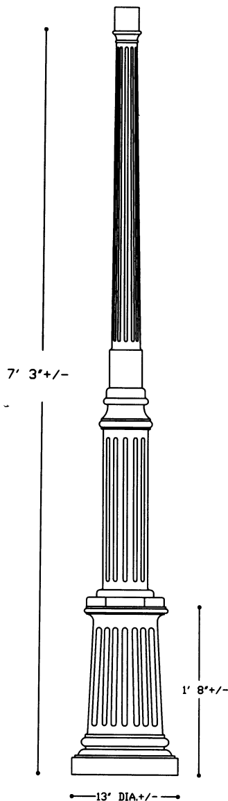
SCALE: 3/4" = 1 FOOT
